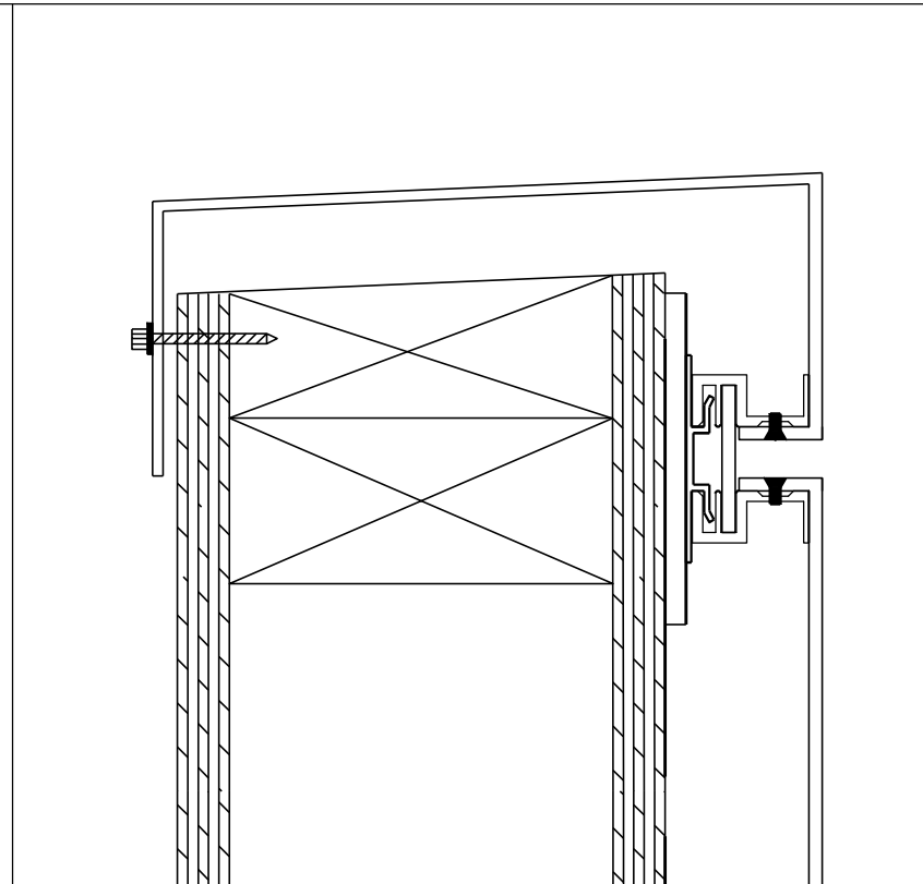
2 310 ACM COPING SCALE: NTS
